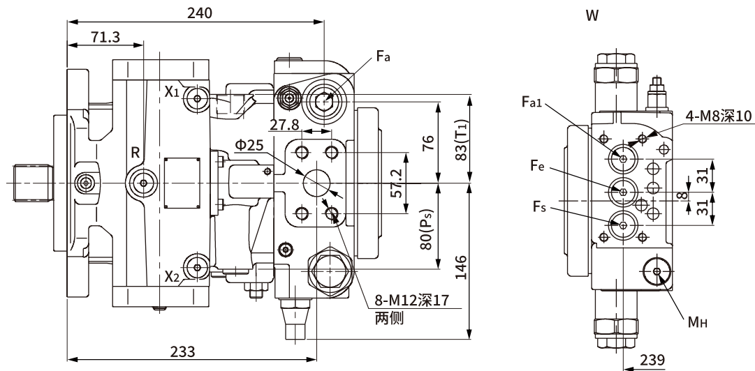
油口DIN3852
