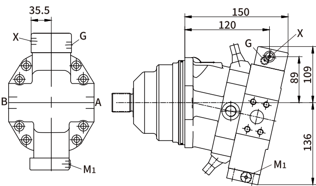
HZ1 两点式液压控制
