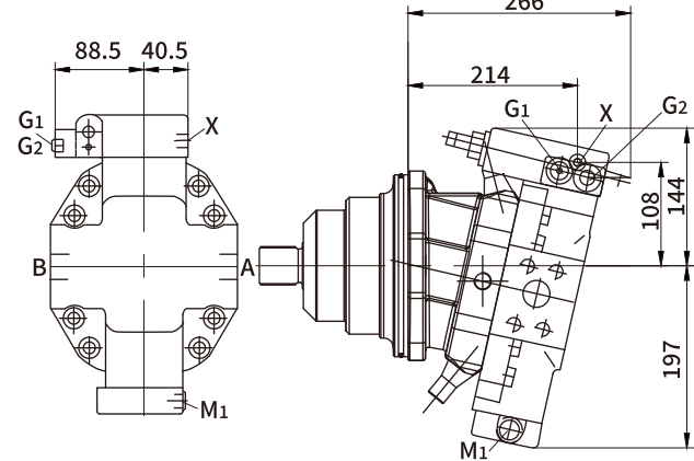
HD.E 压力控制, 两点式液压越权控制
