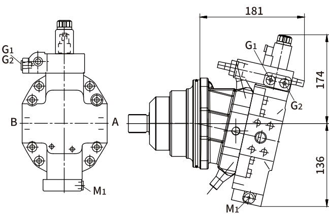
EP.E 电气控制, 两点式液压越权控制
