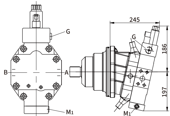
EZ1/EZ2 电气控制, 带开关电磁铁
