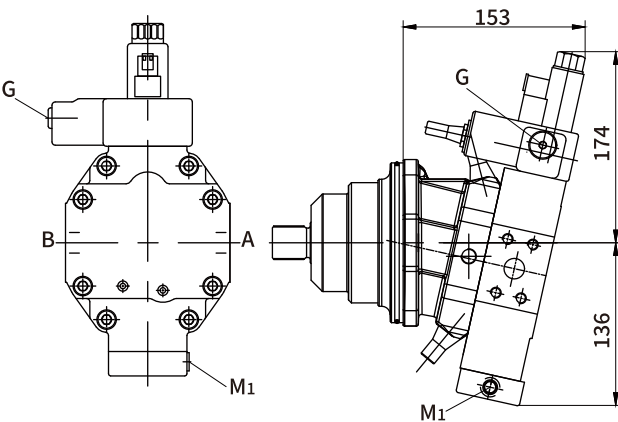
EP.D 电气控制, 固定设置
