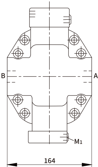
SAE法兰油口A/B在侧面, 相对(02), 仅HZ3/EZ3/EZ4
