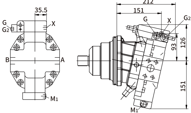
HD.E 压力控制, 两点式液压越权控制
