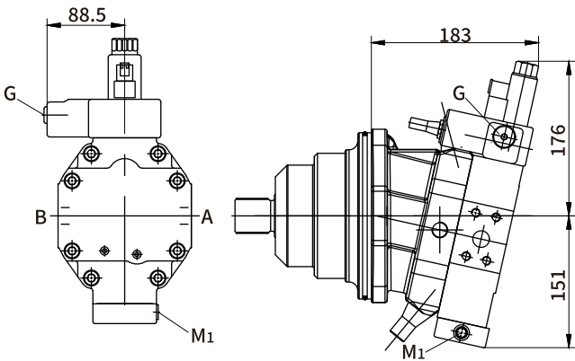
EP.D 电气控制, 固定设置
