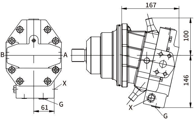
EZ3 两点式液压控制
