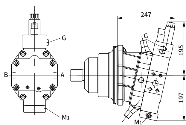
EP1/EP2 电气控制, 带比例电磁铁
