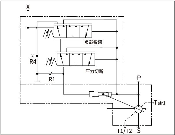
液压回路图
