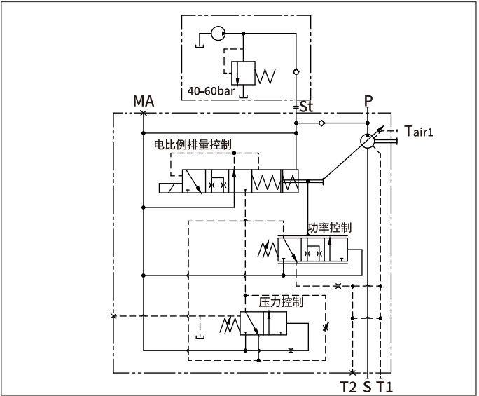
液压回路图
