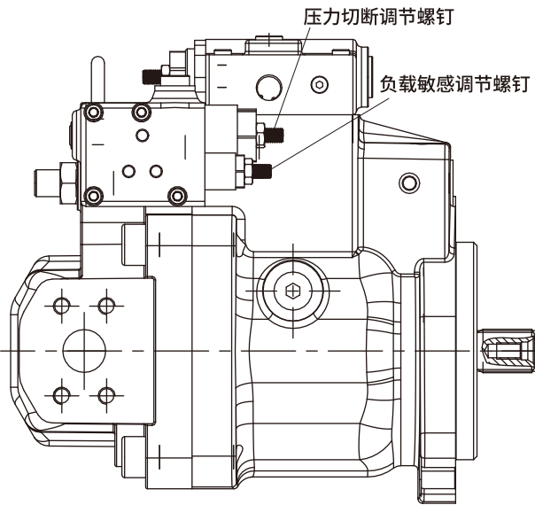
控制阀调节
