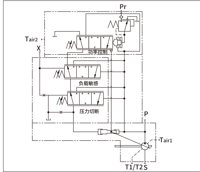
液压回路图
