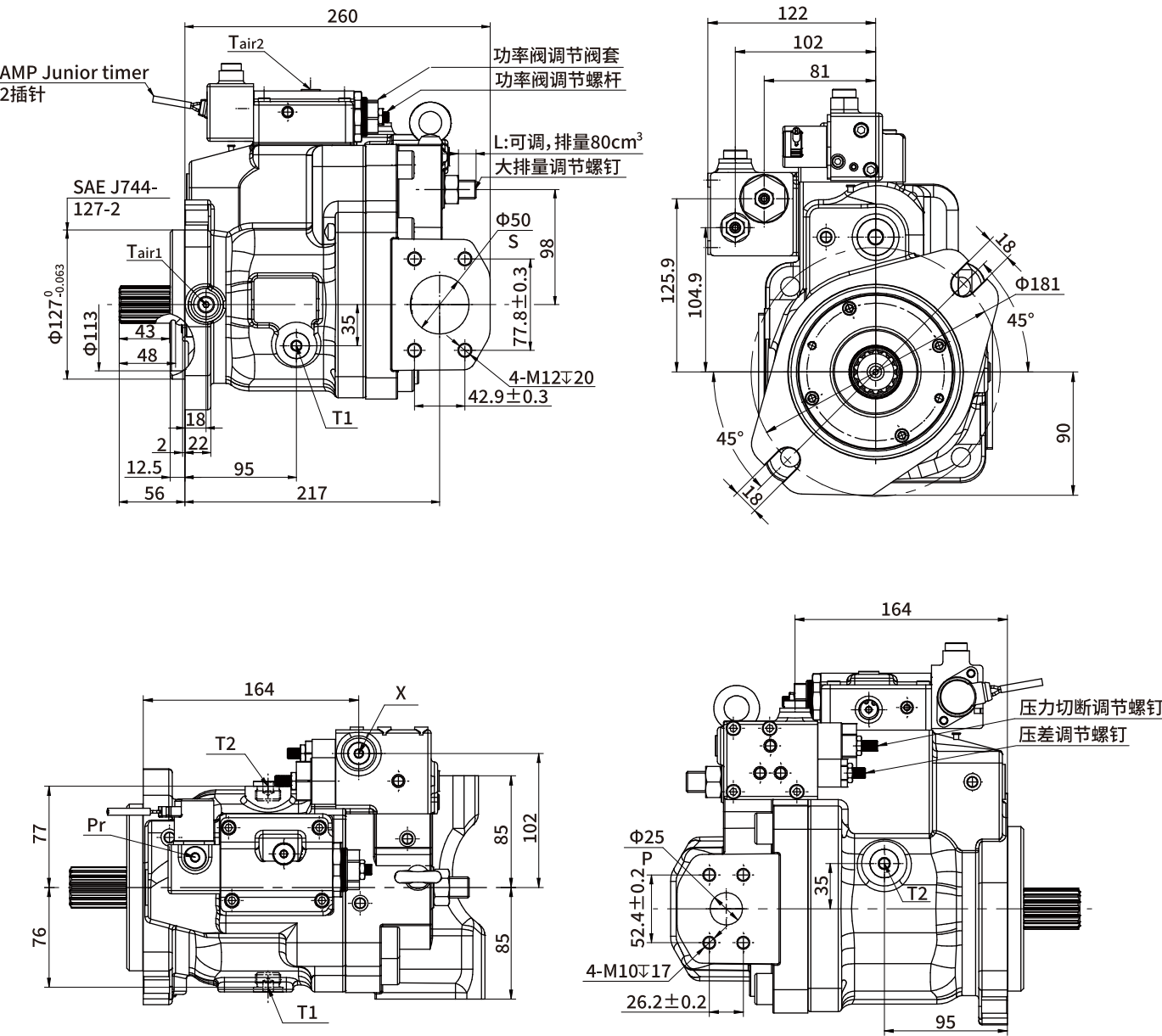
L1/1-E1(L1/1-E2)安装尺寸
