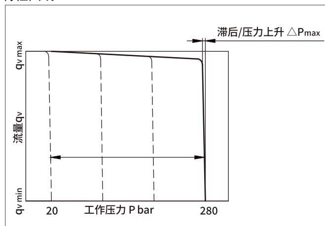
特性曲线
