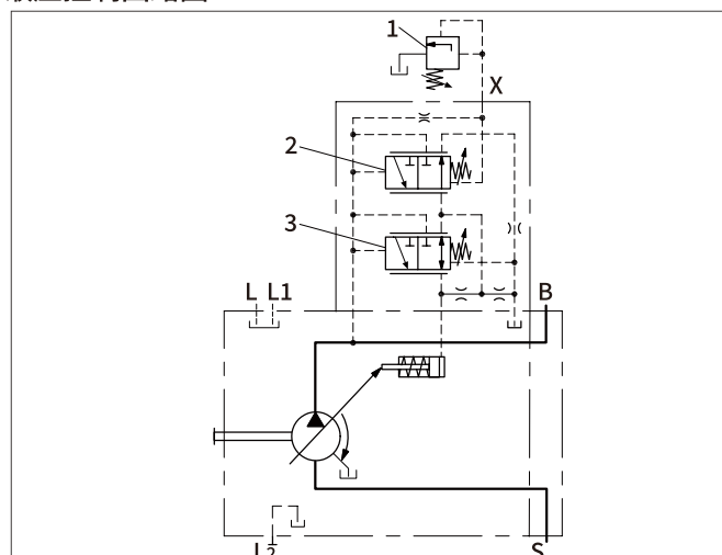
液压控制回路图
