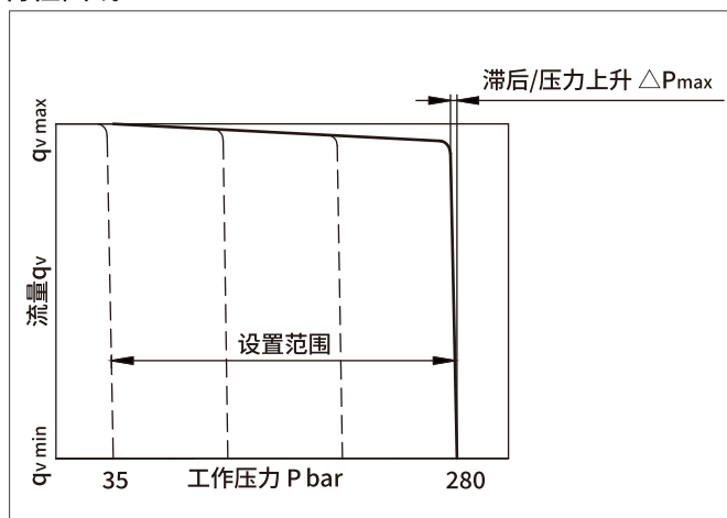
特性曲线
