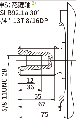
轴伸Z: 花键轴 1) DIN 5480 W50x2x30x24x9g
