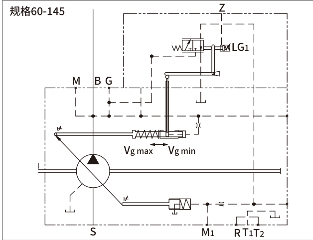
控制原理图
