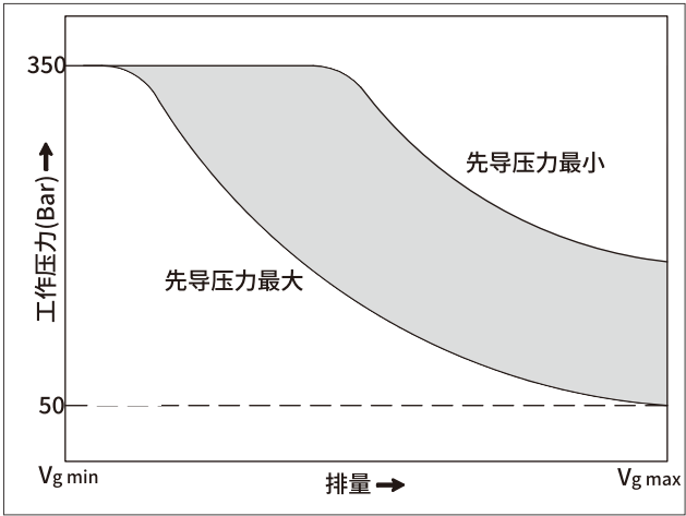
特性曲线
