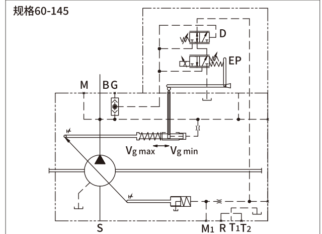
控制原理图
