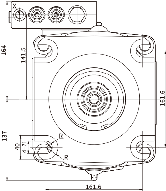
带升压泵 W向
