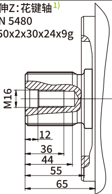
轴伸T: 花键轴 2) ANSI B92.1a 30° 1-3/4" 27T 16/32DP
