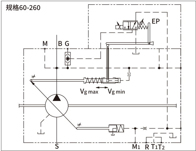
控制原理图
