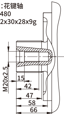
轴伸Z: 花键轴
