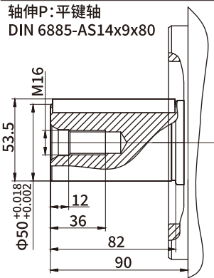
轴伸S: 花键轴 2) ANSI B92.1a 30° 1-3/4" 13T 8/16DP
