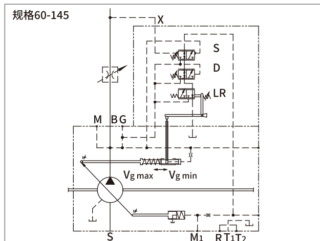
控制原理图
