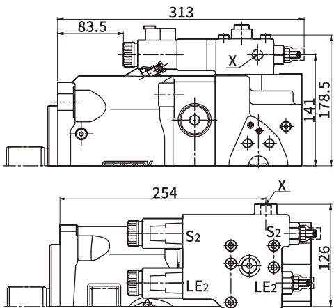
LE2S2 恒功率控制带电子越权 负载敏感控制带电子越权
