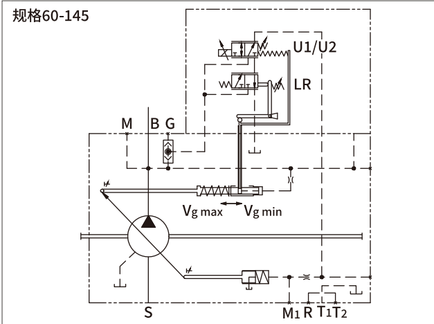
控制原理图
