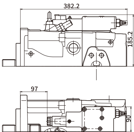
EP2D 带比例电磁铁和压力切断
