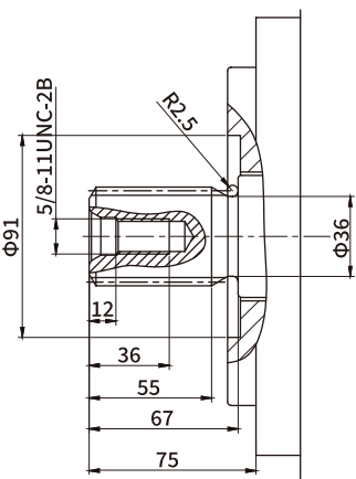
S 花键轴1 3/4" 13T 8/16DP
