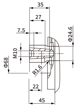
轴伸
