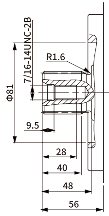
S 花键轴1 1/4" 14T 12/24DP
