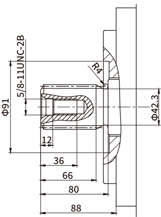
T 花键轴2" 15T 8/16DP
