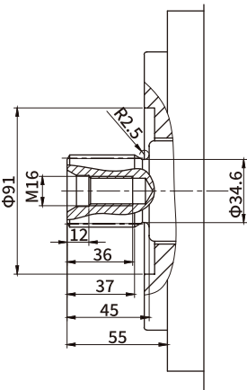
Z 花键轴DIN 5480 W50x2x30x24x9g
