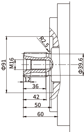
A 花键轴DIN 5480 W70x2x30x22x9g
