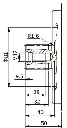
Z 花键轴DIN 5480 W35x2x30x16x9g
