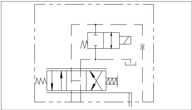
液压原理图, 带常闭式刹车阀, HWC
