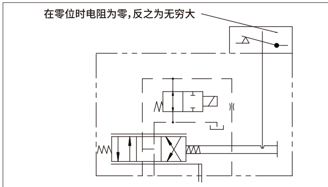
液压原理图, 带常闭式刹车阀和中位开关, HWCL
