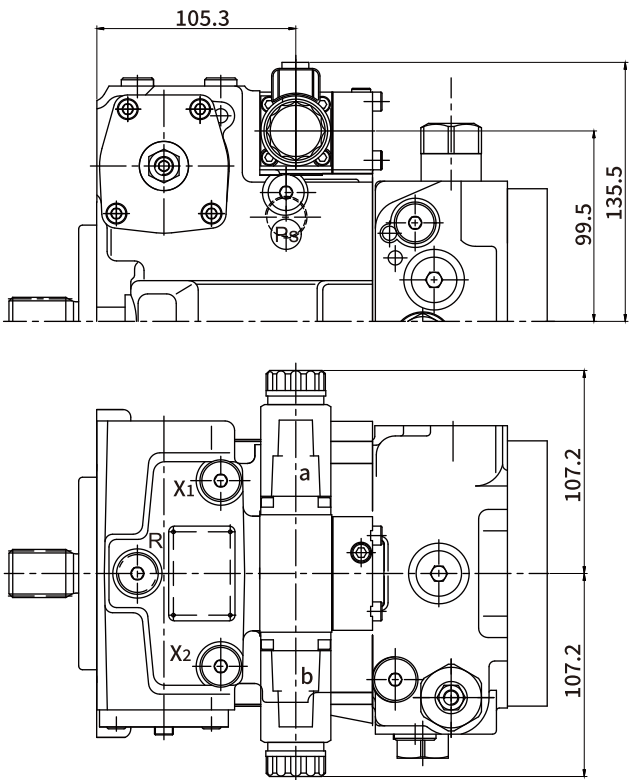
电气控制带比例电磁铁, EP
