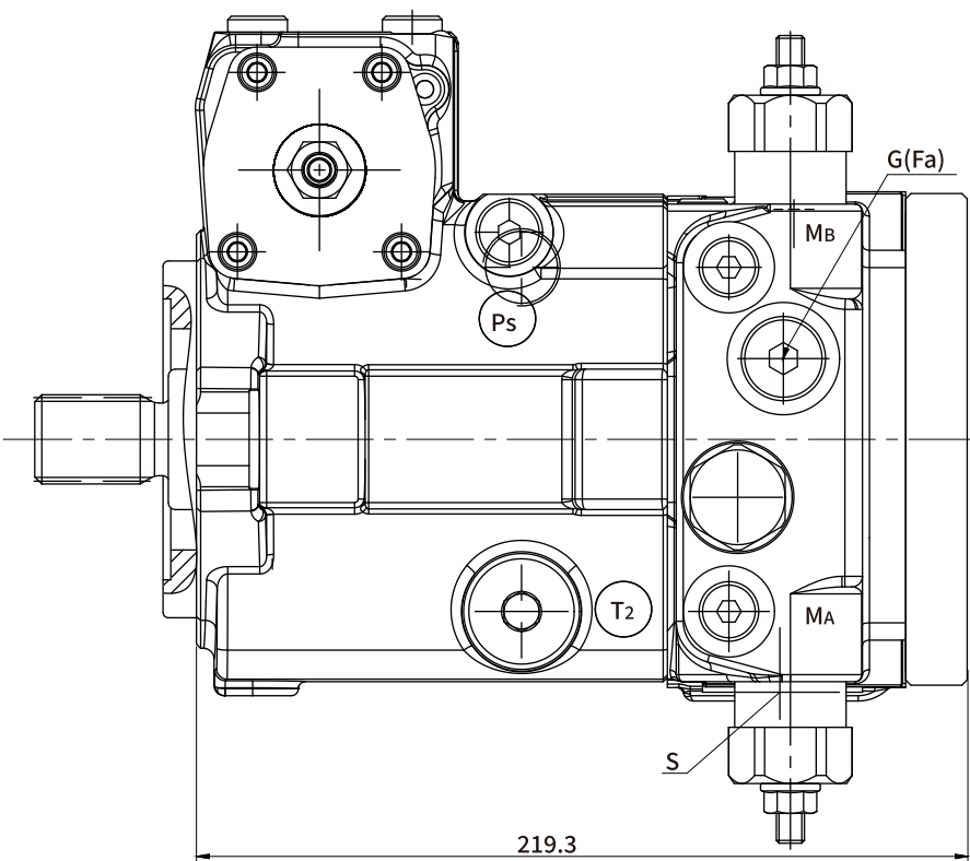
通轴驱动 F01/KO1(5.8mL/r补油泵) 法兰SAE J744-82-2(A)
