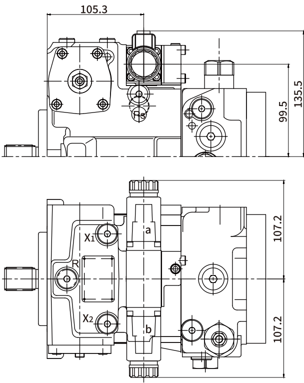
电气控制带开关电磁铁, EZ
