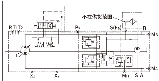
液压原理图-变型二,D
