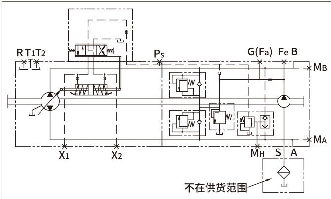
液压原理图-标准型,S
