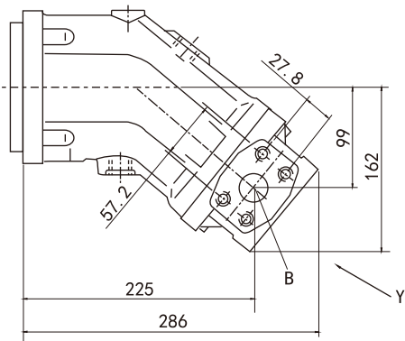
020 SAE 法兰, 在侧面
