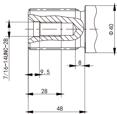
S 花键轴 1 1/4" 14T 12/24DP
