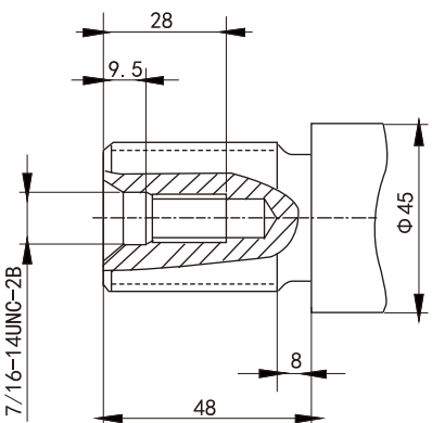
Q 花键轴 1 1/4" 14T 12/24DP
