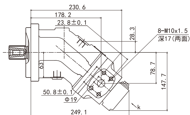
020 SAE 油口法兰, 在侧面
