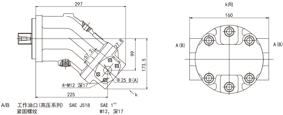
020 SAE 法兰，在侧面
