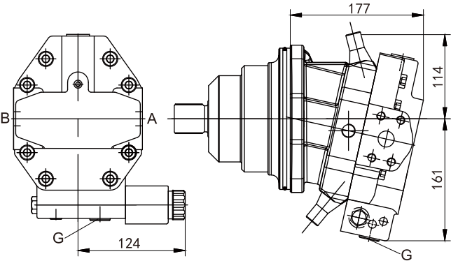
EZ3/EZ4 电气控制，带开关电磁铁
