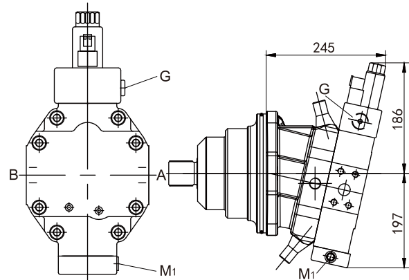
EZ1/EZ2 电气控制，带开关电磁铁
