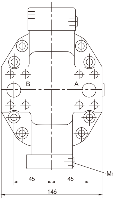
SAE法兰油口A/B在后面，相对(01)
