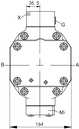
SAE法兰油口A/B在侧面, 相对(02)
