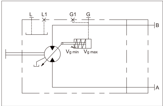
液压原理图，DG
