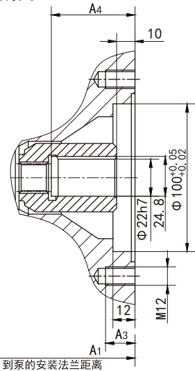
A-B剖面
