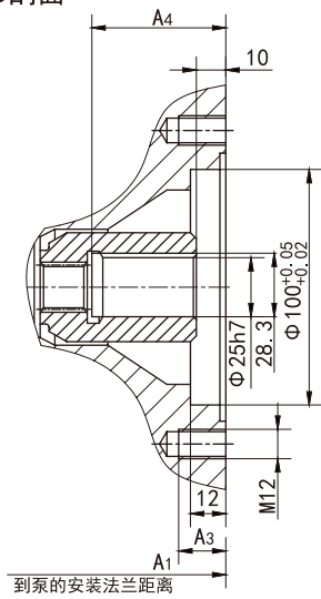
A-B剖面
