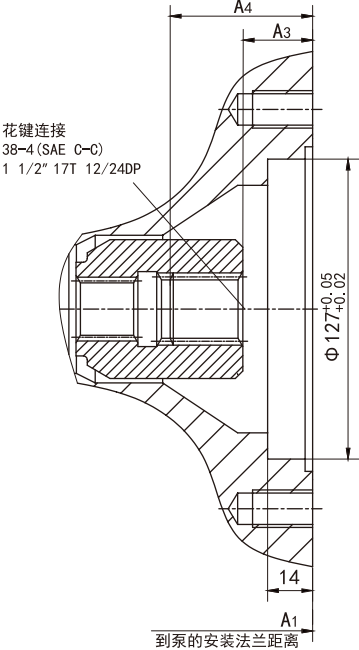
A-B剖面
