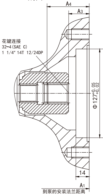
A-B剖面
