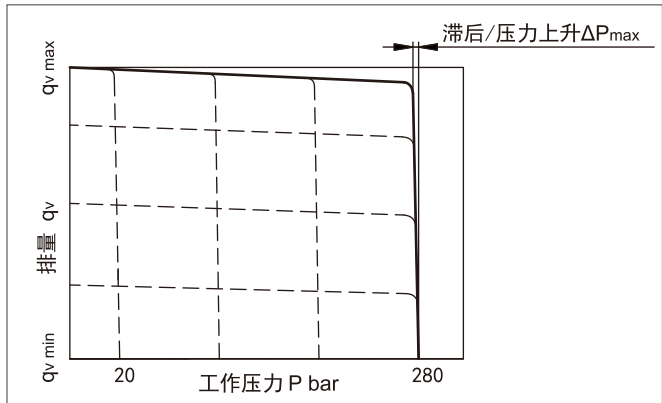
静态工作曲线 (n 1 =1500rpm, t oil =50℃)
