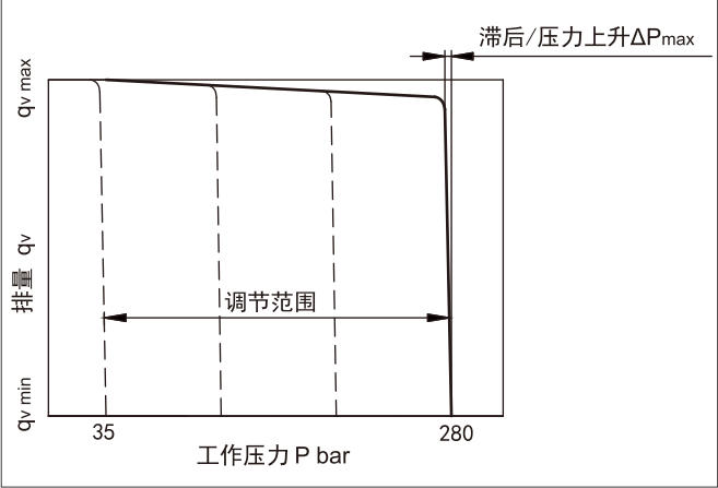
静态工作曲线 (n 1 =1500rpm, t oil =50℃)
