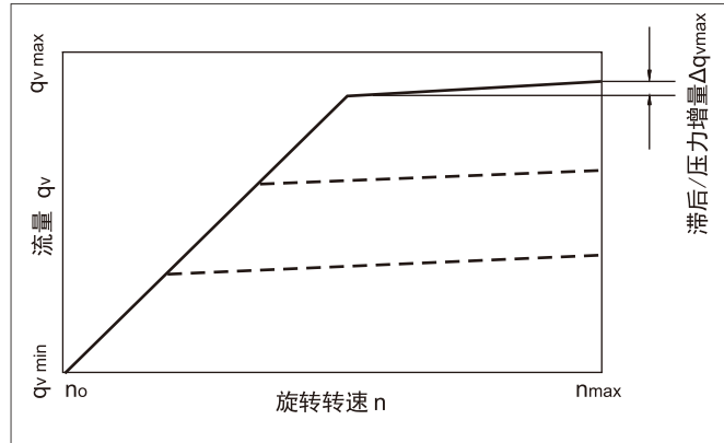
速度变化时工作曲线
