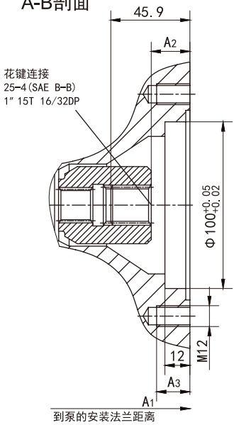
A-B剖面
