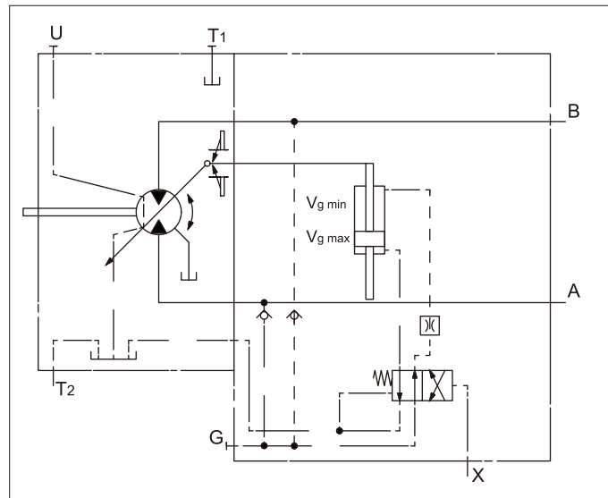
液压控制回路图 HZ3 排量55/80
