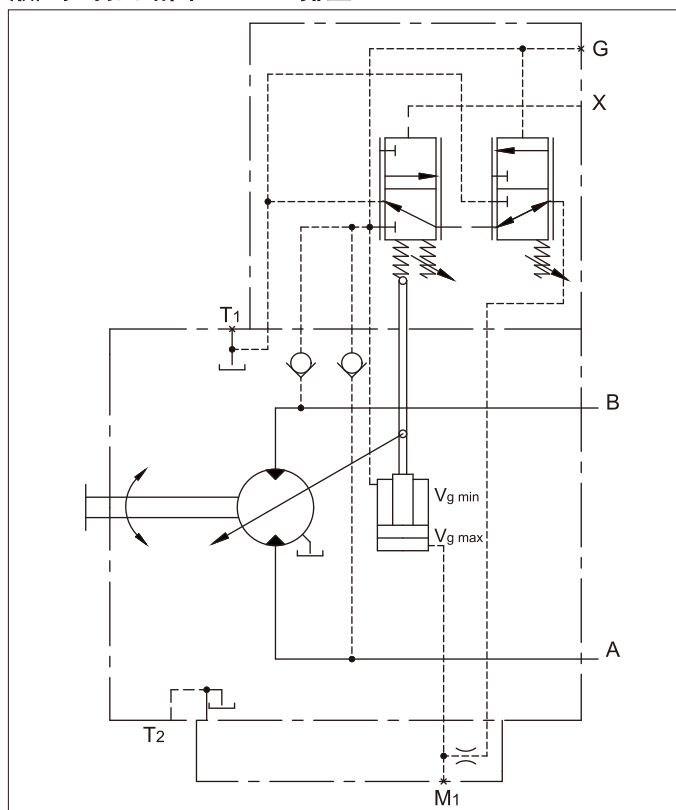
液压控制回路图 HZ1.D 排量107-200
