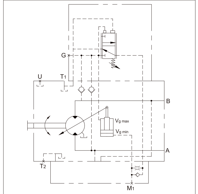
液压控制回路图 HA1
