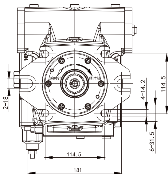
六孔法兰
