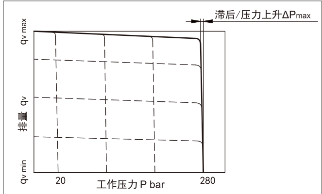
静态工作曲线 (n 1 =1500rpm, t oil =50℃)
