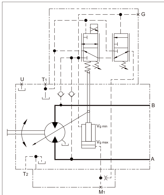
液压控制回路图 EP.D
