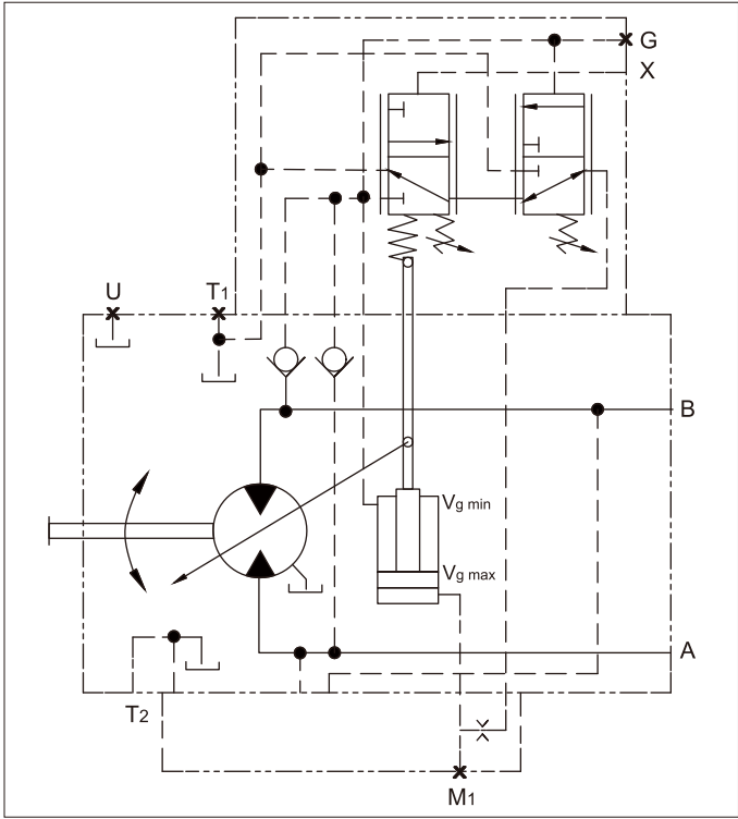
液压控制回路图 HD.D 排量28-200
