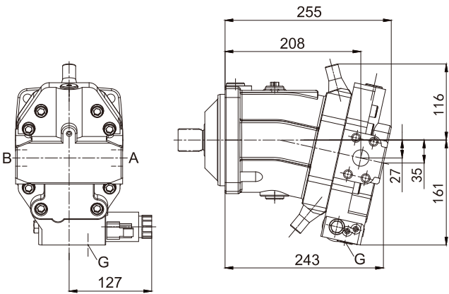
EZ3/EZ4 电气控制, 带开关电磁铁
