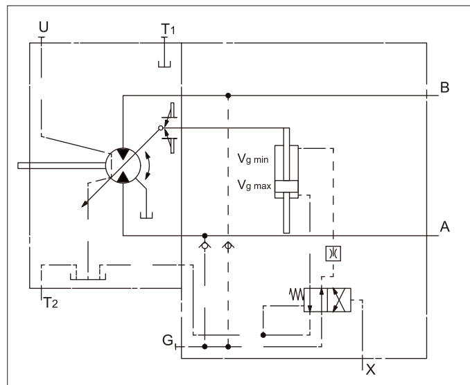
液压控制回路图 HZ3 排量55/80
