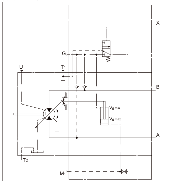
液压控制回路图 HZ1 排量28/107/115/130/160/170/200
