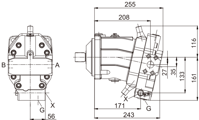
HZ3 两点式液压控制
