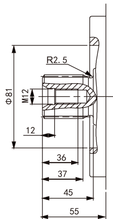
A 花键轴 DIN 5480 W40x2x30x18x9g
