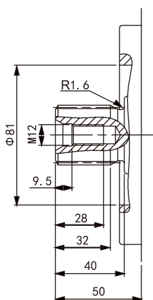
Z 花键轴 DIN 5480 W35x2x30x16x9g
