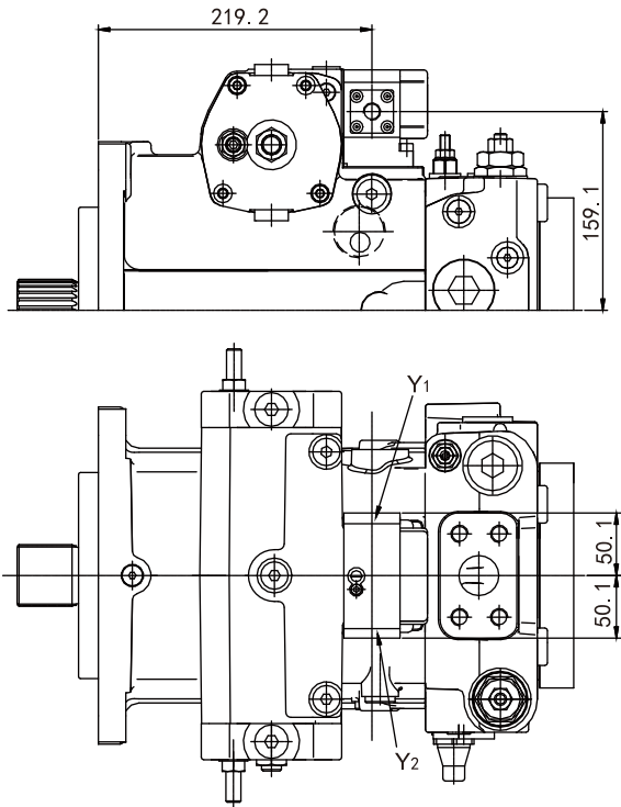
Y1/Y2 远程控制油口 M14x1.5 深12
