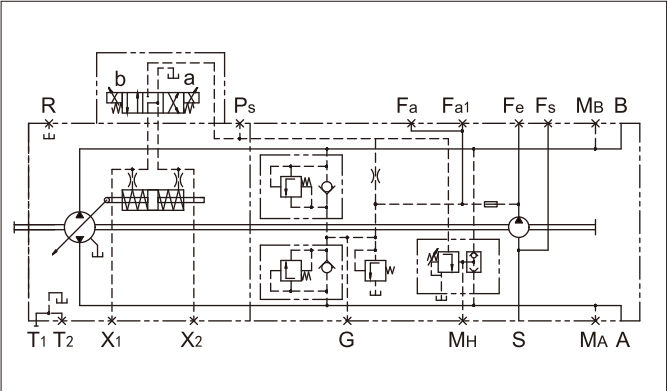
液压原理图
