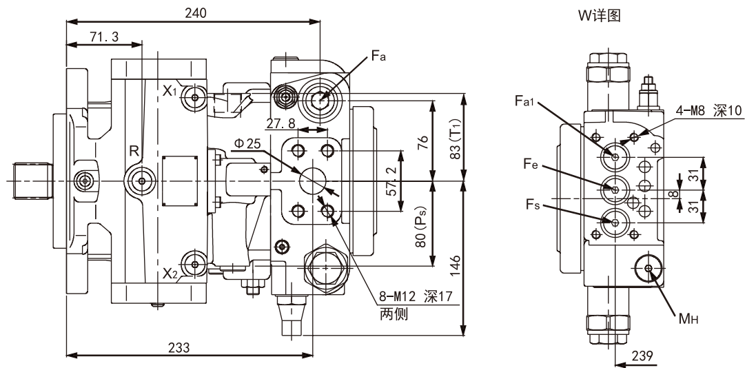
油口 DIN3852
