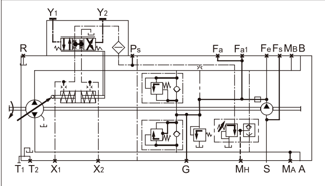
液压原理图，HD3
