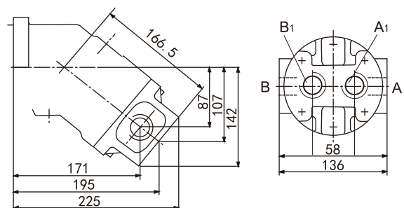
04 螺纹油口，在侧面和后面
