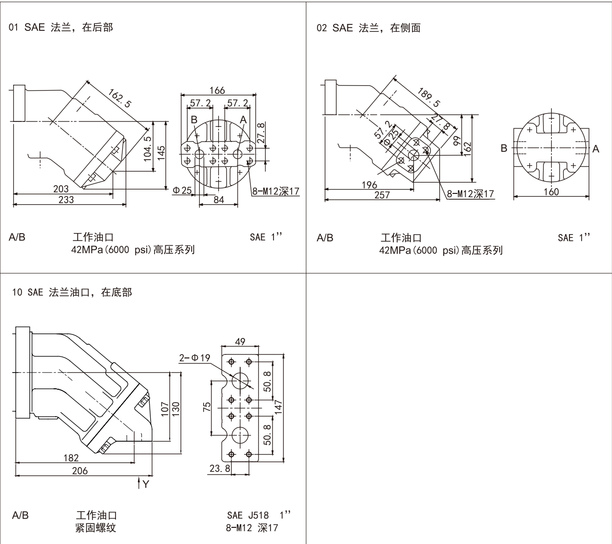
油口接板
