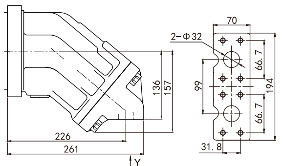
10 SAE 法兰油口，在底部
