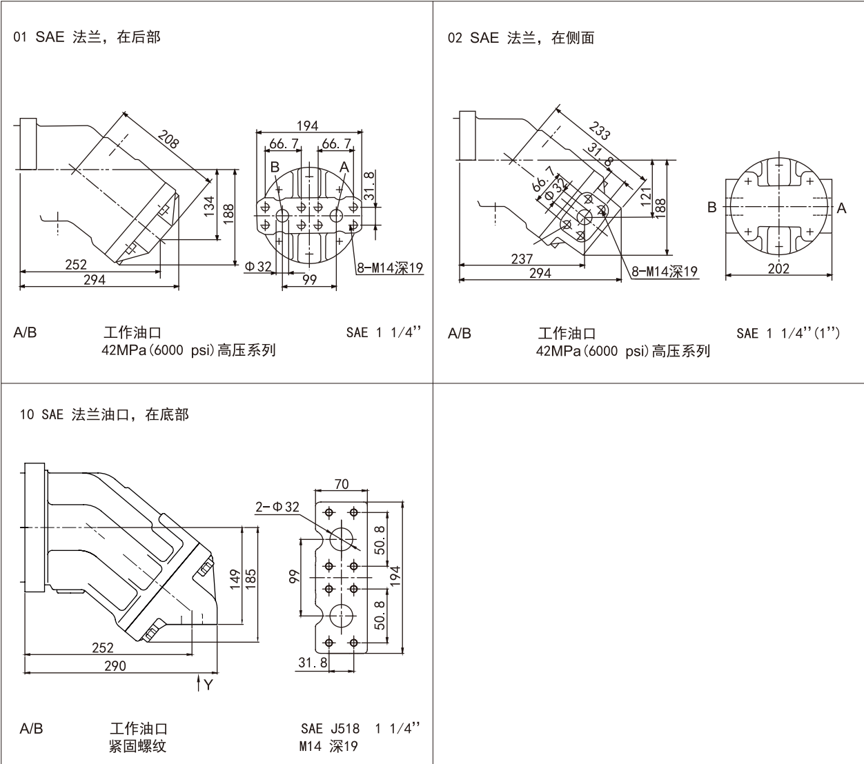
油口接板
