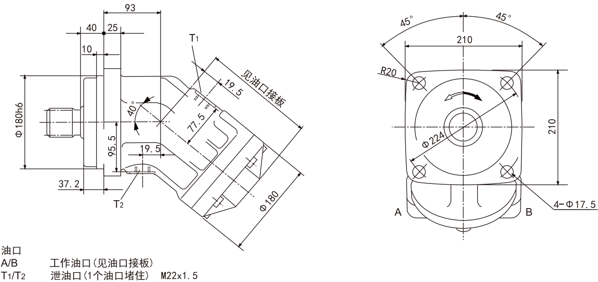
HA2FM 160/180
