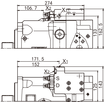
DRS 压力控制 带负载敏感控制
