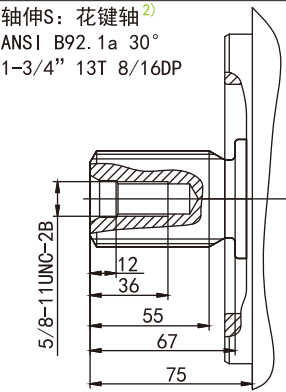
轴伸Z: 花键轴 1) DIN 5480 W50x2x30x24x9g
