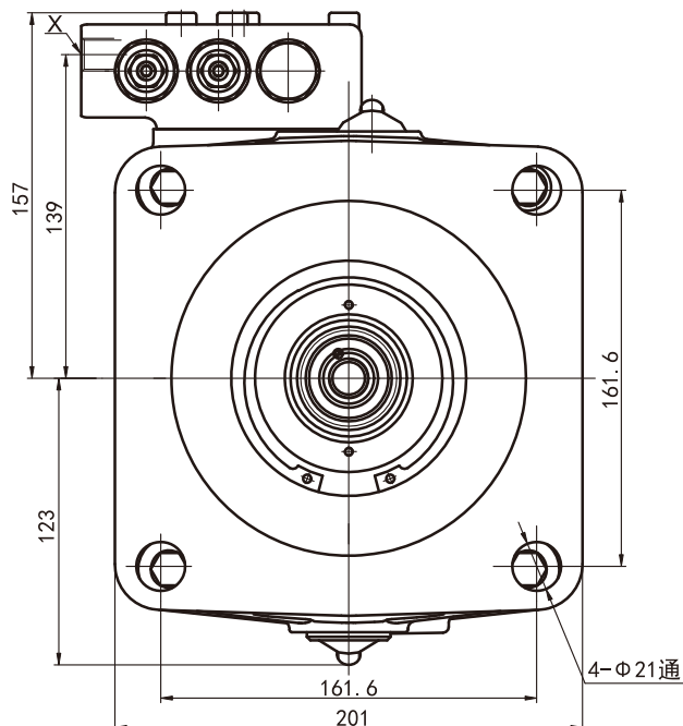
W向 287 234 4-M16深24 \Phi 75 S 106.4 61.9 V向 287 234 4-M12深17 \Phi 25 B 57.2 27.8
