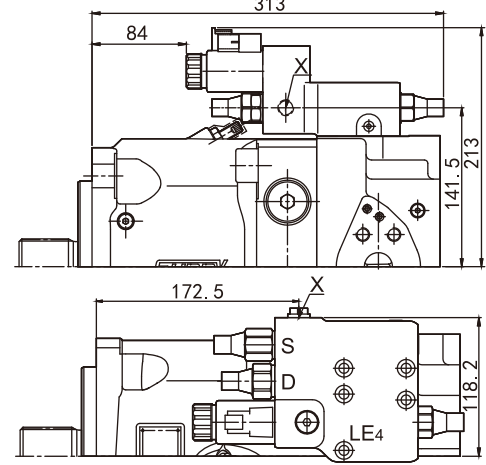
LE4DS 恒功率控制带电子越权 带压力控制和负载敏感控制
