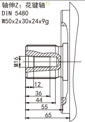
轴伸T: 花键轴 2) ANSI B92.1a 30° 1-3/4" 27T 16/32DP
